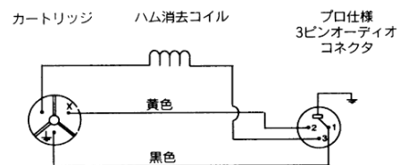
内部接続図
