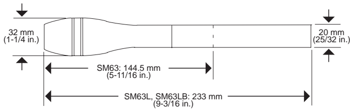
DIMENSIONES GENERALES
